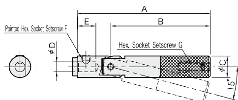
QLTL-RL (Plug-In Handles)
